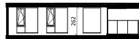
Doorsnede loft 1:200
