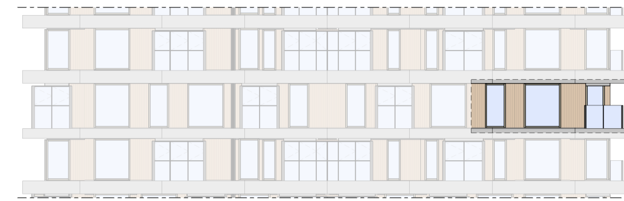
Westgevel 1:200
