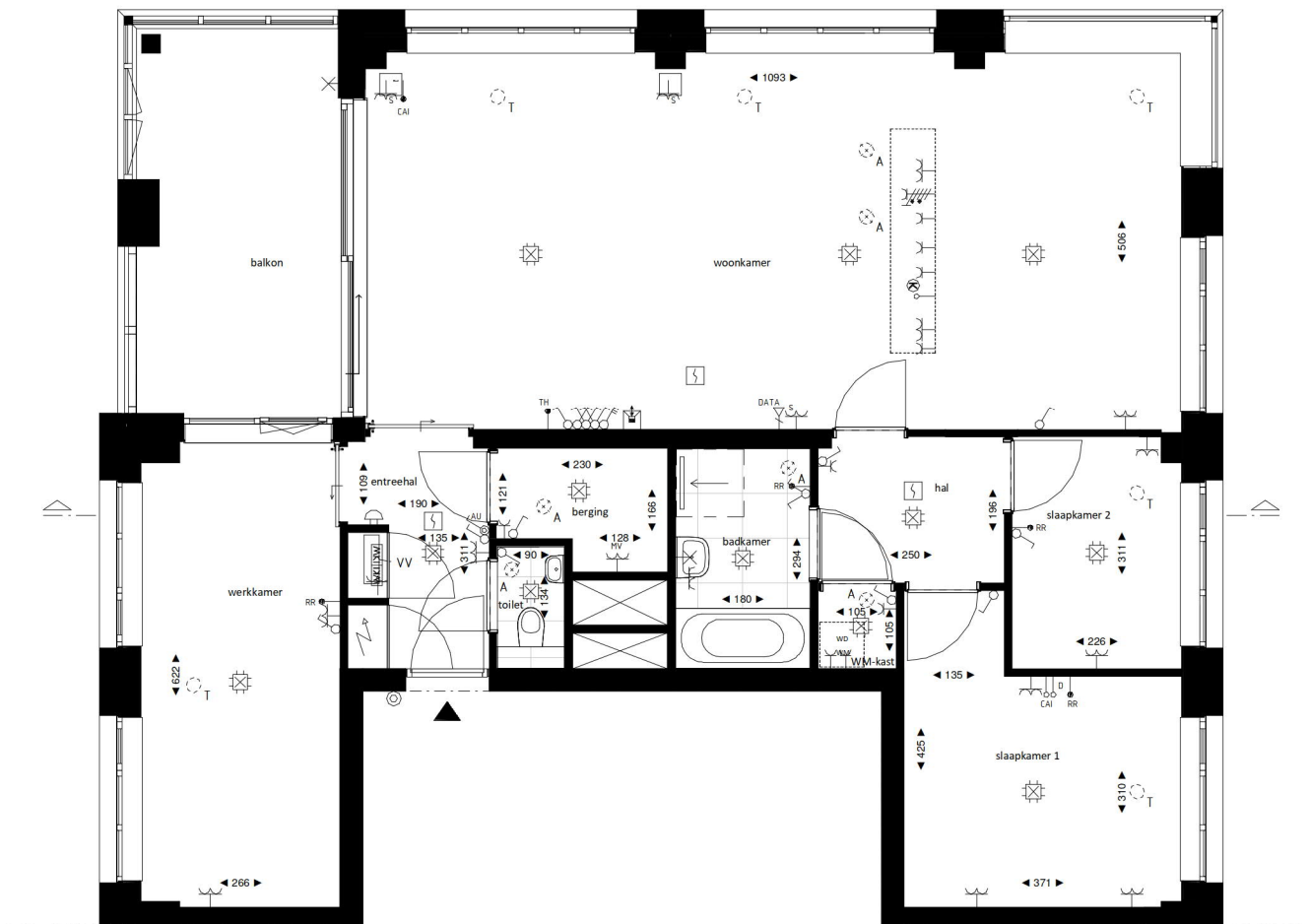
Loft 1:50
