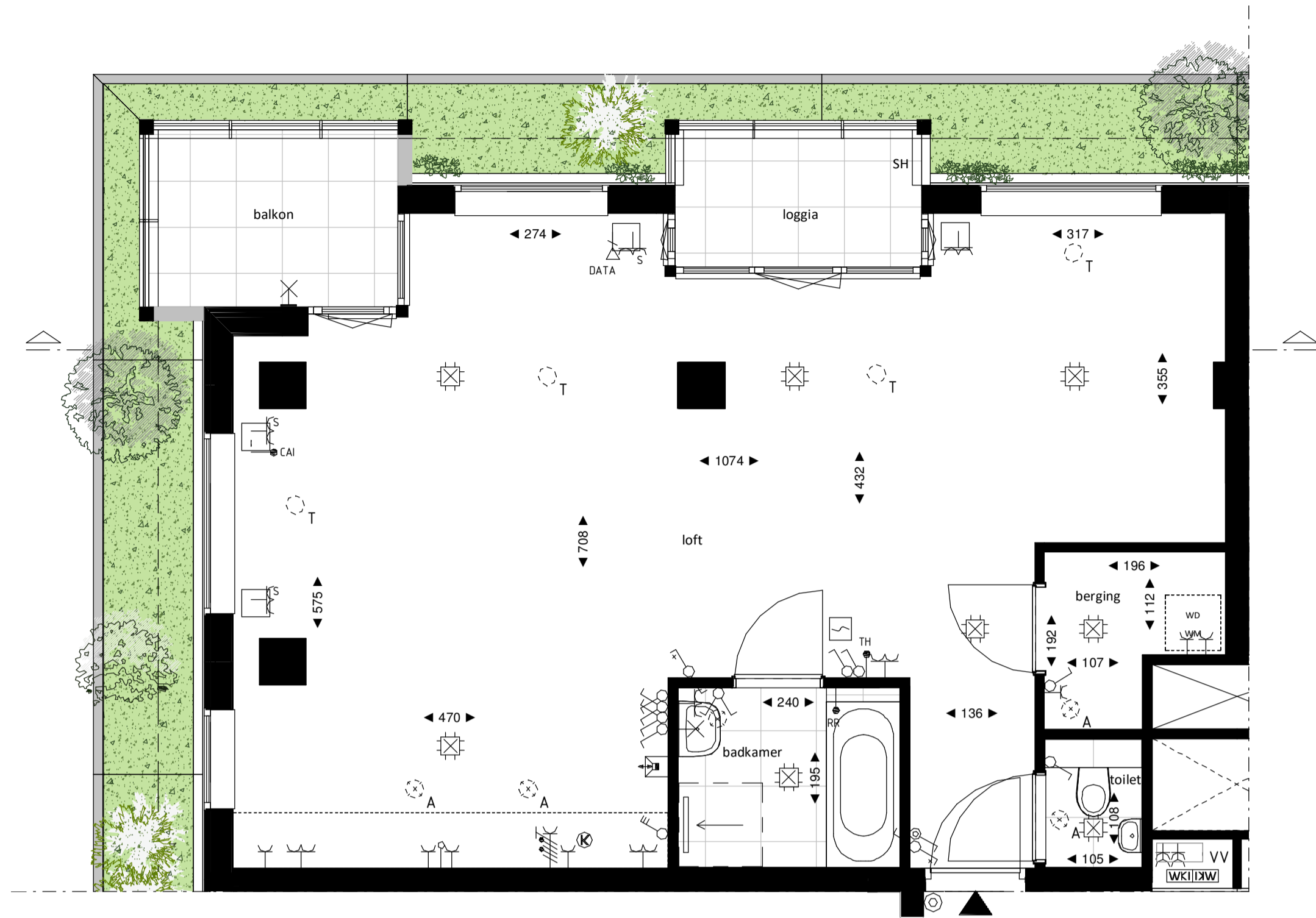
Loft 1 : 50
