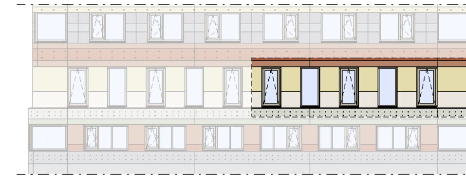
Oostgevel 1:200
