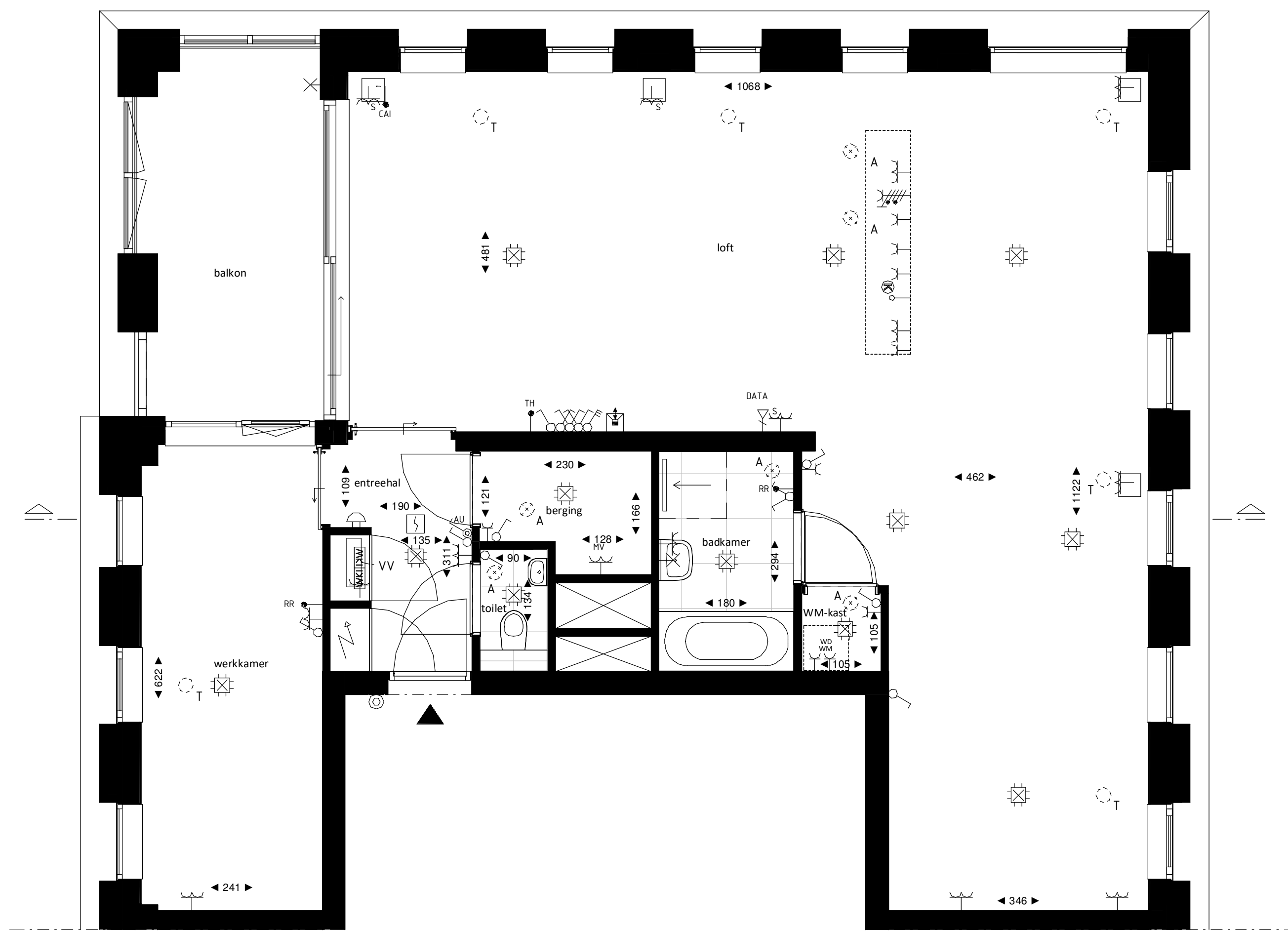
Loft 1:50
