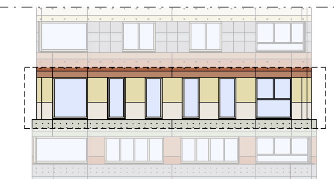
Noordgevel 1:200
