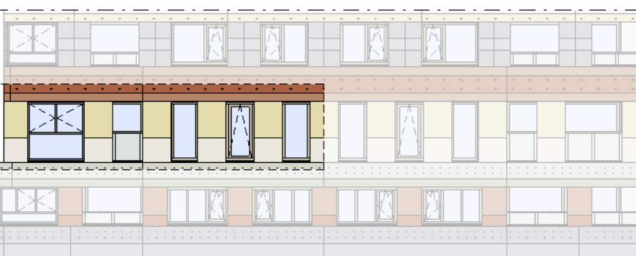
Westgevel 1:200
