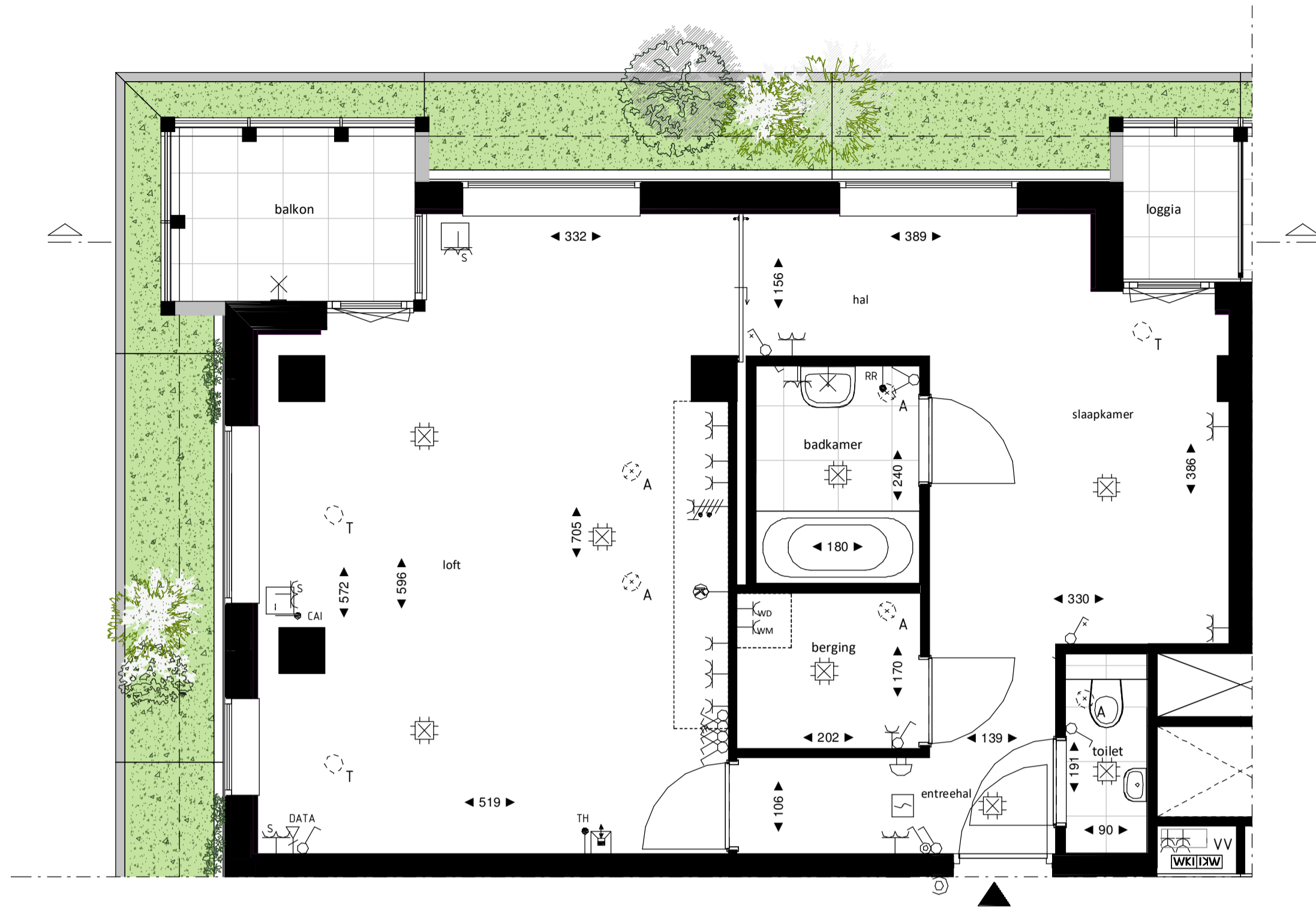
Loft 1 : 50
