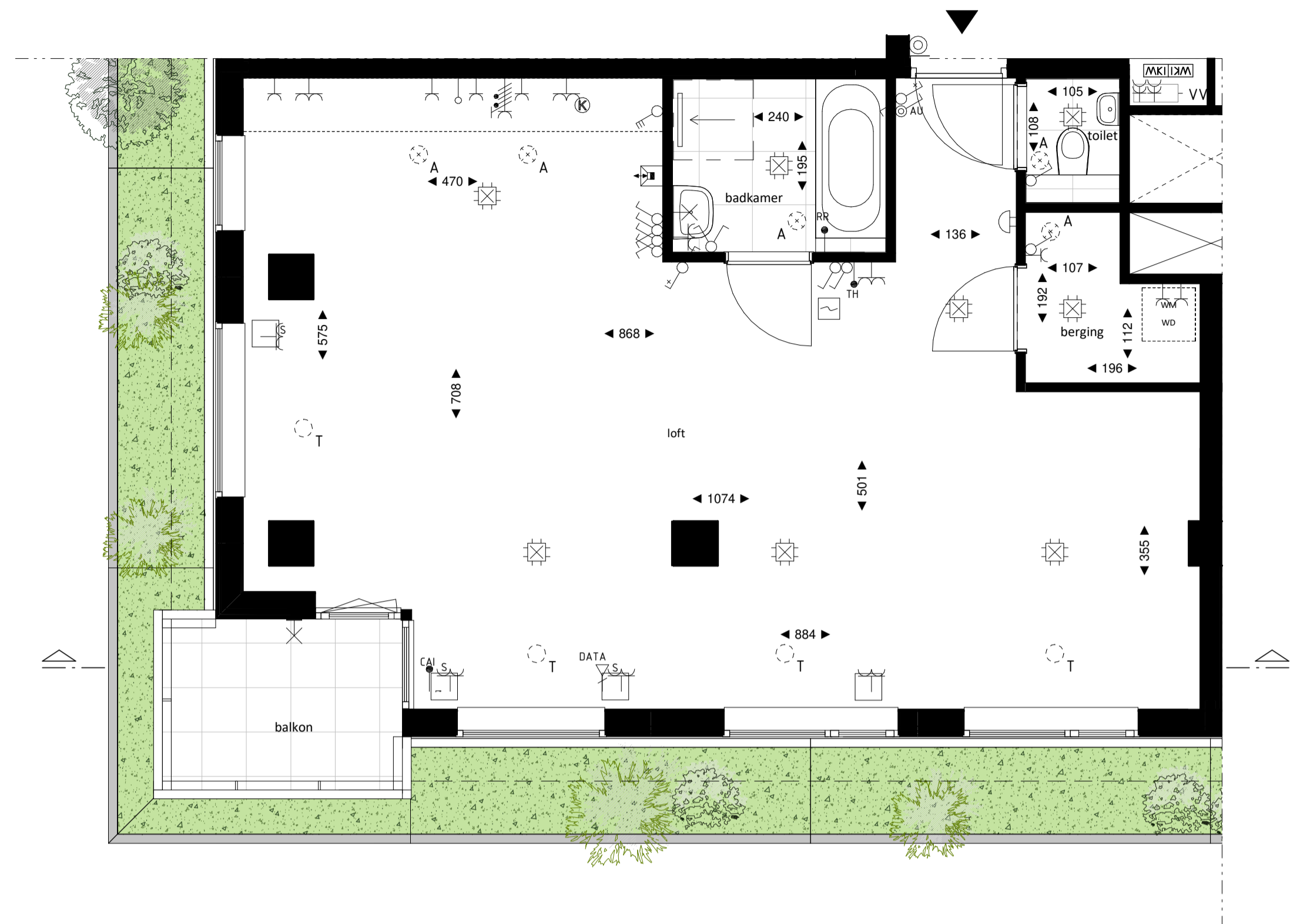
Loft 1:50
