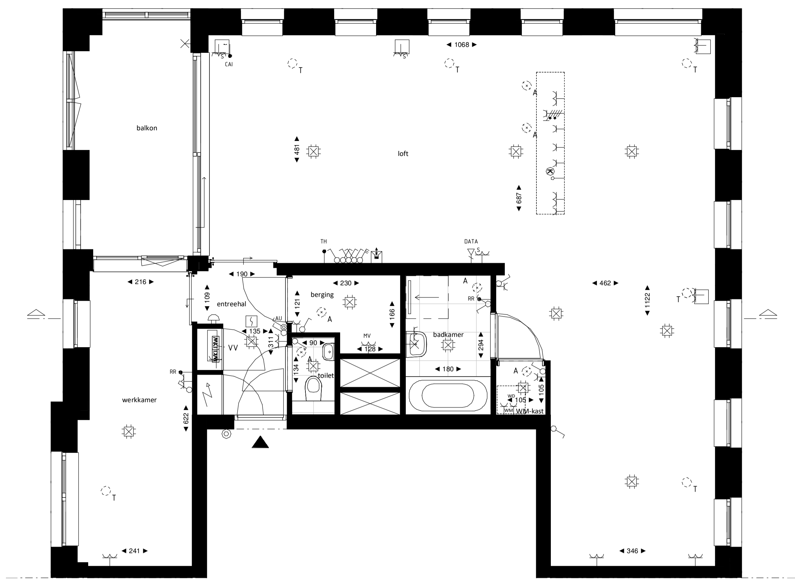
Loft 1:50
