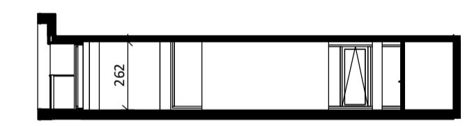
Doorsnede loft 1:200
