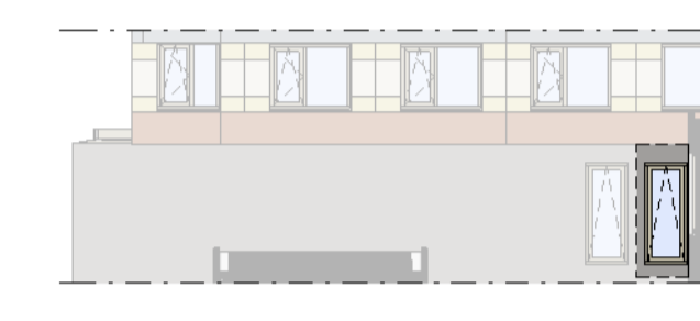
Oostgevel 1:200
