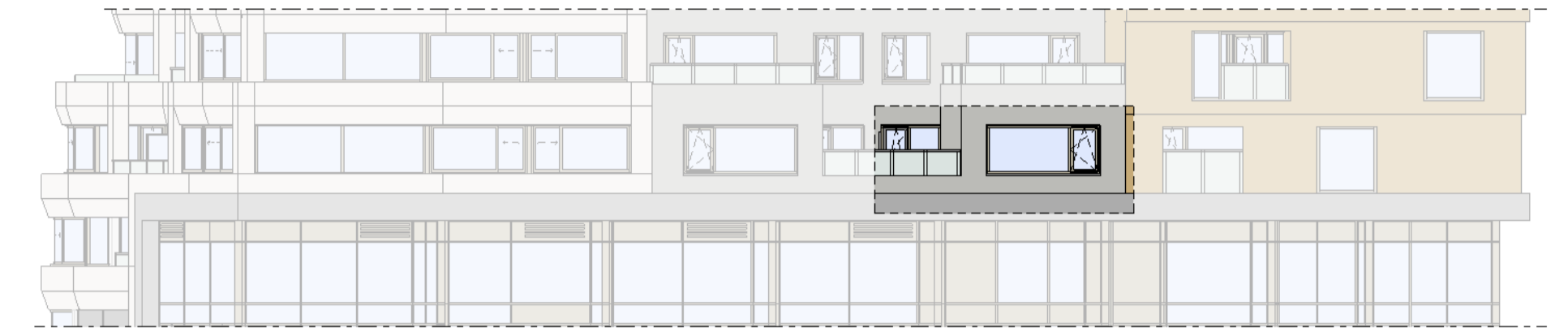
Oostgevel 1 : 200
